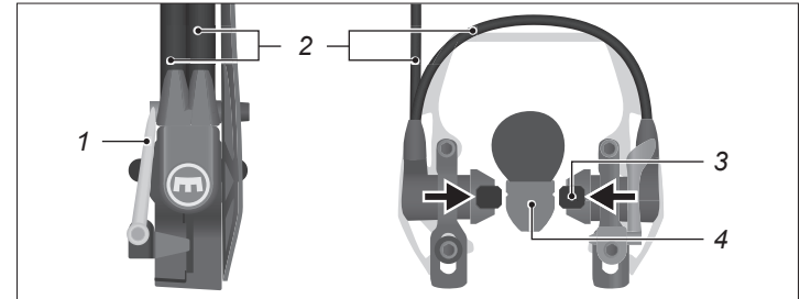
Abb. Hydraulische Felgenbremse
