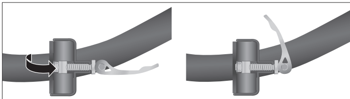
Abb.: Klappverschluss mit Spannhebel schließen
