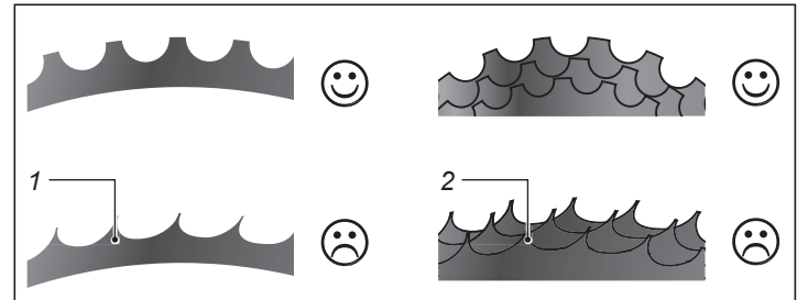
Abb.: Zahnkranz
